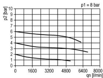
Diagramă de debit
