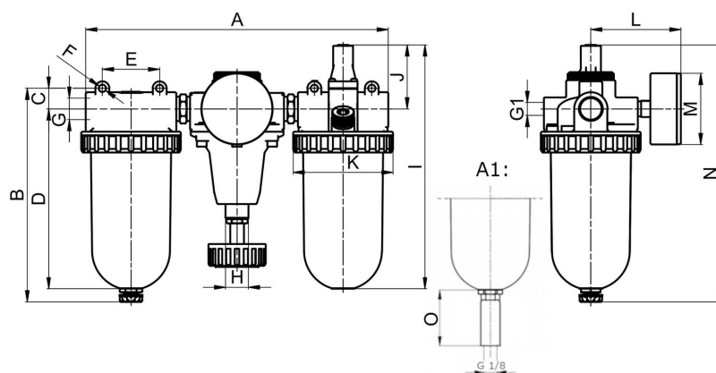
A1: automatisch aftapventiel
