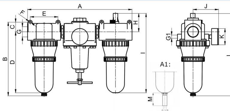
A1: automatisk aftapningsventil
