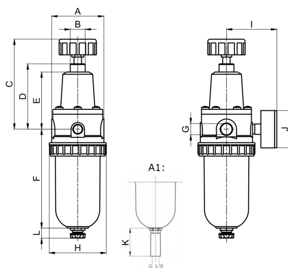
A1: automatisk aftapningsventil
