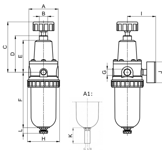
A1: supapă de purjare automată
