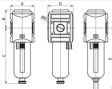
puoliautomaattinen tyhjennysventtiili
