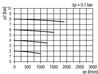
FI18-38H/12-F0,01
