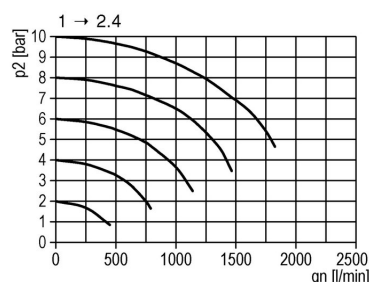
2. Virtauskaavio
