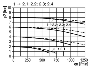
2. Virtauskaavio
