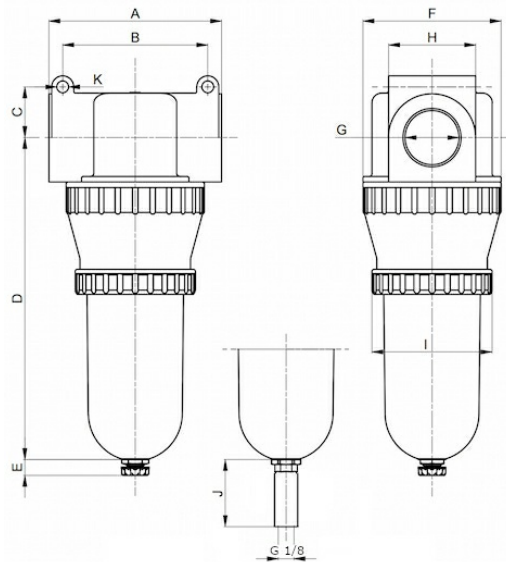
purgeur automatique
