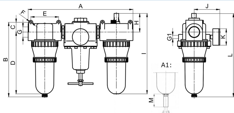
A1: αυτόματη βαλβίδα αποστράγγισης
