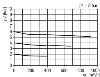
Strømningsdiagramm
