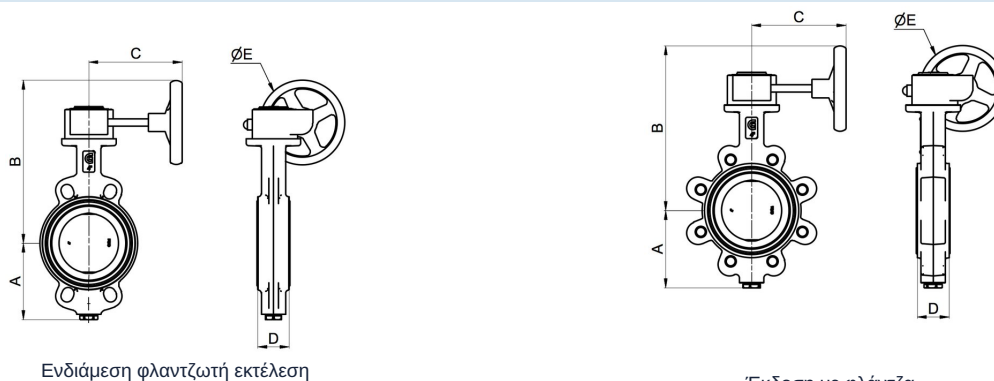
Έκδοση με φλάντζα
