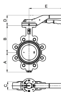
Laippaliitännäversio
