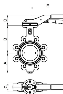
Prirubnička izvedba
