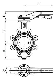
Versione flangiata
