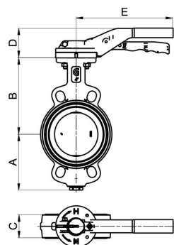
Execuție cu flanșă intermediară
