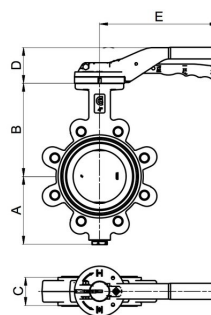
Execuție cu flanșă
