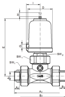
Fjäder stänger
