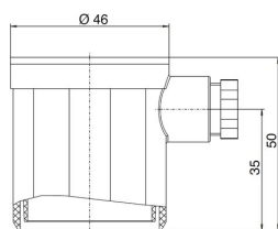
Beskyttelseshætte med PG-forskruing Type 6371 (IP54) / 6372 (IP65)
