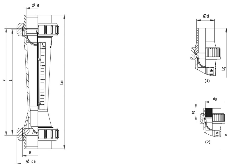
(1)...Priključak s nastavkom za zavarivanje, (2)...Priključak s navojnom čahurom
