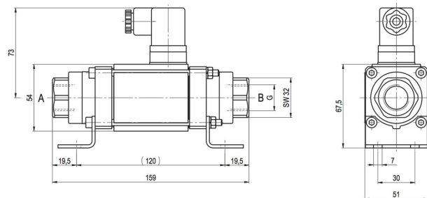
CVT-10 Functie NO
