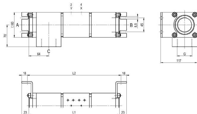
CVTV3-40 Fonction NC
