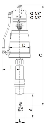
Regulator de poziție P/P Tip 8047
