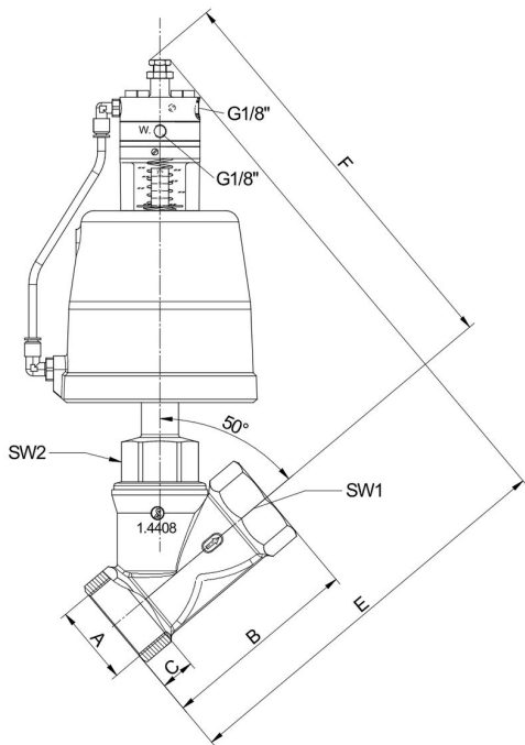
p/p-Stellungsregler Typ 8047
