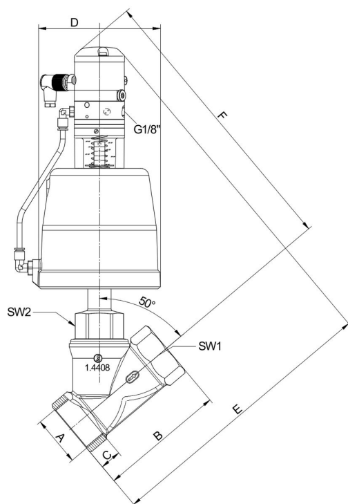
i/p-Stellungsregler Typ 8047
