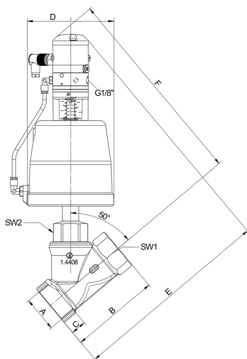
i/p-Stellungsregler Typ 8047
