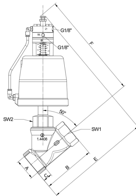
p/p-Stellungsregler Typ 8047
