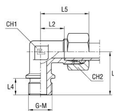
B3-vágógyűrűvel
